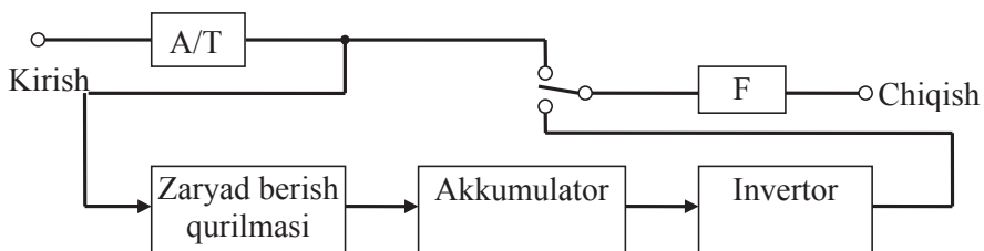
11.7-rasm. Chiziqli-interfaol UPS sxemasi.
