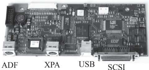
4.14-rasm. Interfeysli plata (SCSI- va USB-portlarni muvofiqalashtiradi hamda qo'shimcha modullarni ulash uchun ikkita razyom qismiga ega).
