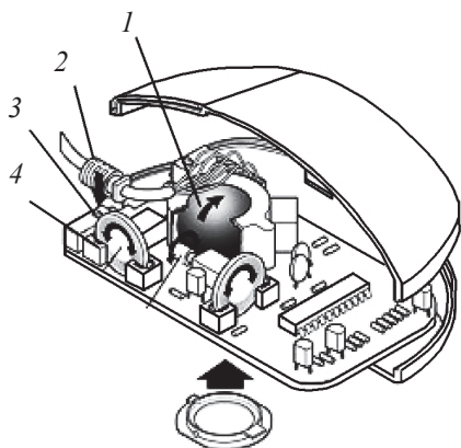
4.2-rasm. Optik mexanik sichqoncha mexanizmi: 1 – qo‘l harakati yo‘nalishi bo‘yicha sichqoncha harakatlanadi; 2 – sichqonchani tizim bilan ulash interfeysi; 3 – buyruqlarni tanlash yoki uzatish tugmalari; 4 – vertikal va gorizontal aylantirish roliklari.
