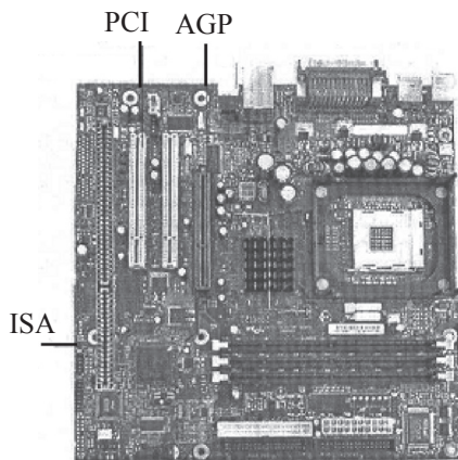
8.7-rasm. Kompyuterning tizimli platasidagi slotlarning joylashuvi.
