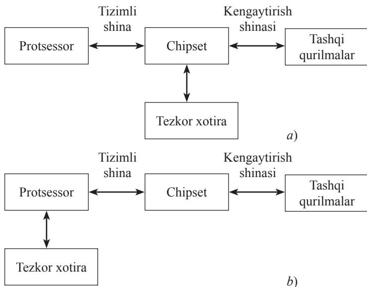
2.3-rasm. Tizimli plataning ishlash tamoyili:
