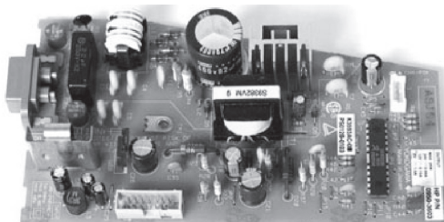
4.15-rasm. Skanerning elektr ta'minot bloki o'rnatilgan plata.
