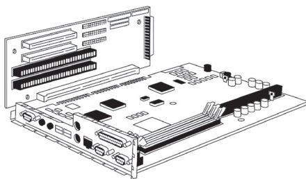
2.6-rasm. NLX standartining tizimli platasi.
