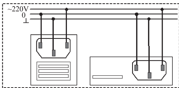
11.2-rasm. Ikki qurilmani elektr ta'minoti zanjiriga ulash varianti.
