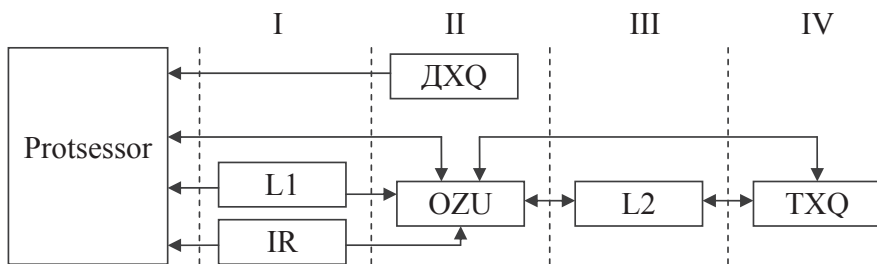
1.3-rasm. Mikroprotsessor xotirasining turlari va pogʻonalar sxemasi.
