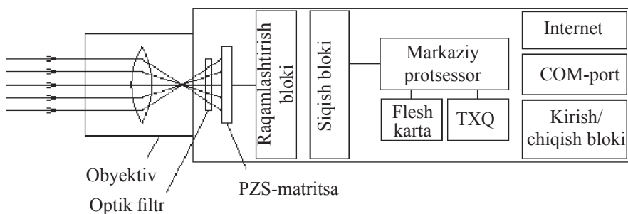
7.15-rasm. Web-kameraning komponentlari.
