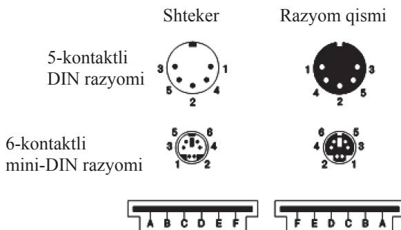
4.4-rasm. Klaviatura va sichqonchanning razyomi.
