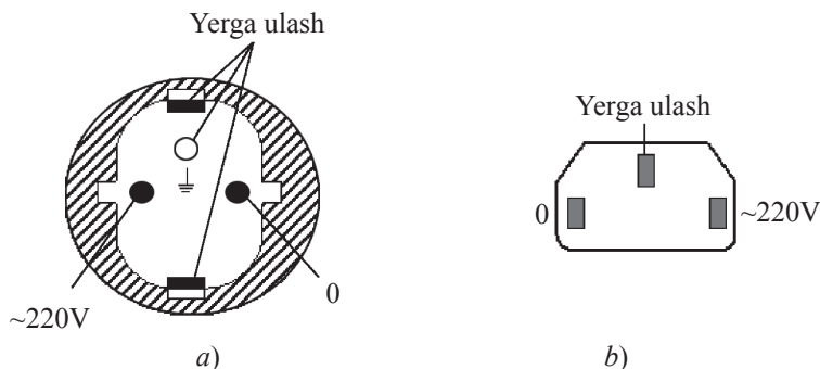
11.3-rasm. Rozetkadagi kontaktlarning to‘g‘ri holati.
