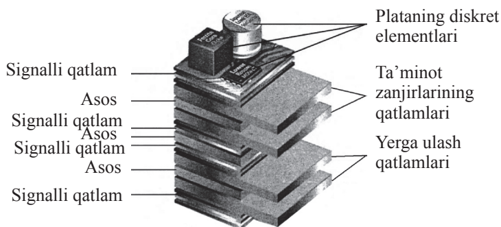
2.2-rasm. Tizimli plata qatlamlari.
