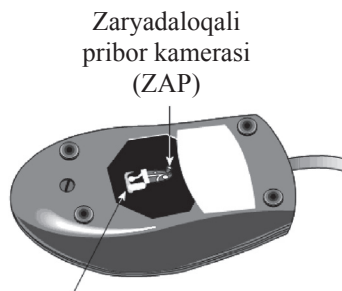
Zaryadaloqali pribor kamerasi (ZAP) Yorug‘lik tarqatuvchi diod (YTD) yuzani yoritishda foydalaniladi
