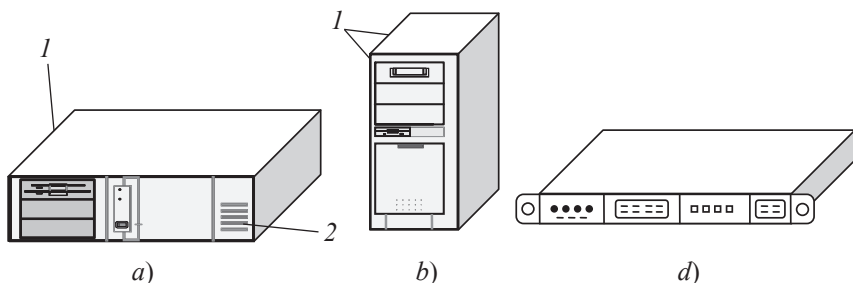
1.4-rasm. Tizimli blokning konstruksiyasi.
