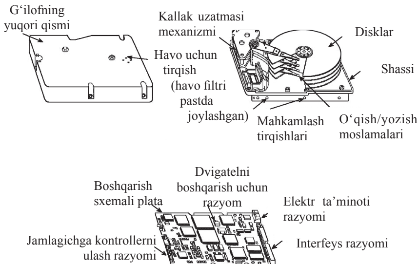
3.1-rasm. Qattiq diskdagi jamlagichlarning asosiy bog‘lamalari.
