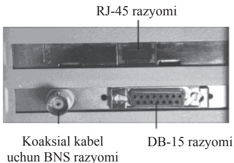
8.6-rasm. Ethernet razyomlari.
