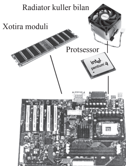
2.1-rasm. Tizimli plataga o‘rnatiladigan elementlar.
