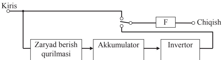
11.6-rasm. Off-Line tipidagi UPS sxemasi.
